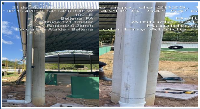
FOTO 13: ITEM 8.5 - FIXAÇÃO DE TUBOS VERTICAIS DE PPR DIÂMETROS MAIORES QUE 75 MM COM ABRAÇADEIRA METÁLICA RÍGIDA TIPO D 3", FIXADA EM PERFILADO EM ALVENARIA. AF_05/2015
