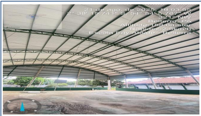
FOTO 02: ITEM 6.4.1 - Cobertura - telha em aço galvanizado e=0,5mm
